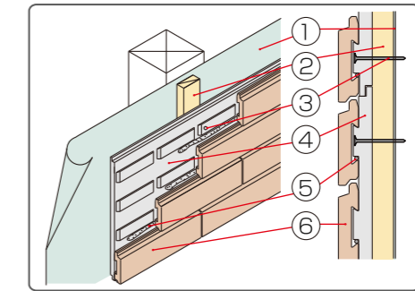
[木造(木軸)構成図](ブリックタイプ)
