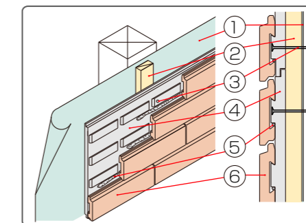
[木造(木軸)構成図](ブリックタイプ)
