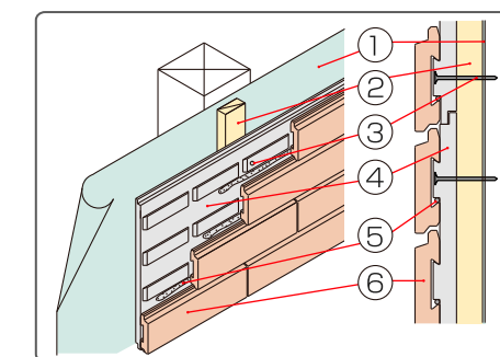
[木造(木軸)構成図](ブリックタイプ)
