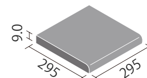
段鼻形状
