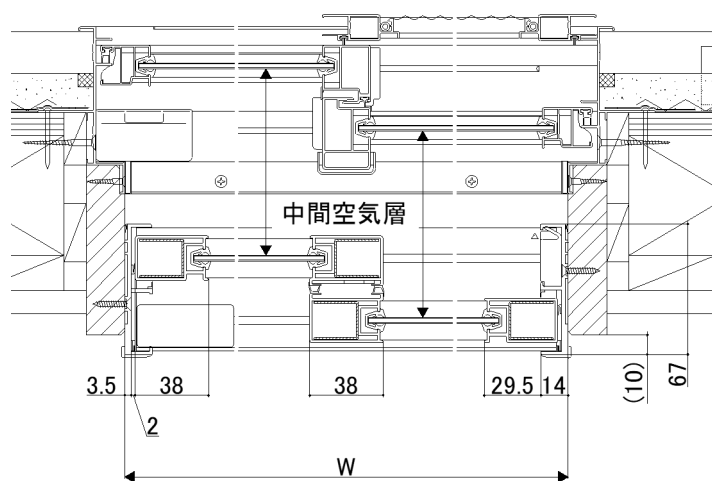
4枚建合掌部
