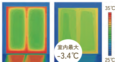
シェードなし シェードあり 夏期における室内表面温度※2
