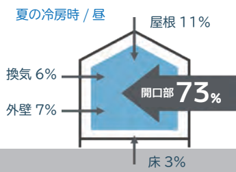
室外の熱が室内に入り込む割合
